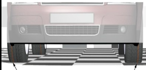
כוון סמני סטיית גלגול הצמיגים הקדמיים מנוגדים, הרכב יתמיד במסלולו.
